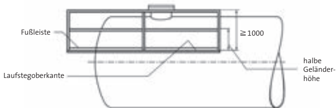
Arbeitsbühne mit freistehendem Geländer, z.B. bei Chemikalienfahrzeugen
