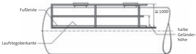
Laufsteg mit feststehendem Geländer
