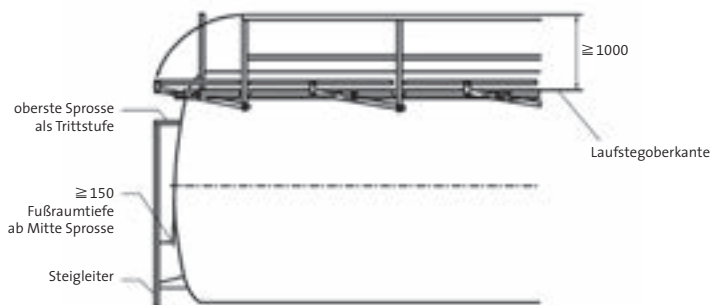
Geländer parallel zum Laufsteg klappbar
