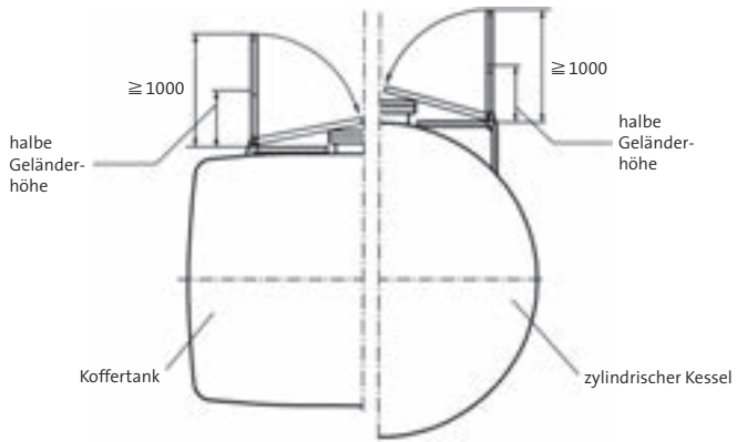
Seitlich klappbares Geländer
