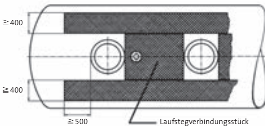
Doppelter Laufsteg mit Verbindungsstück
