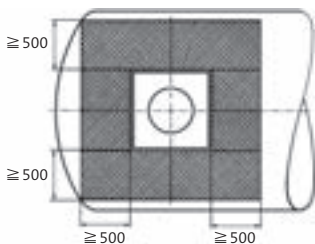
Arbeitsbühne für einen Dom
