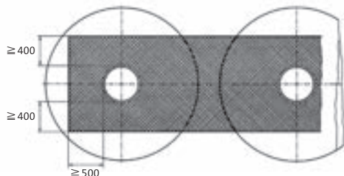
Arbeitsfläche bei mehreren stehenden Behältern
